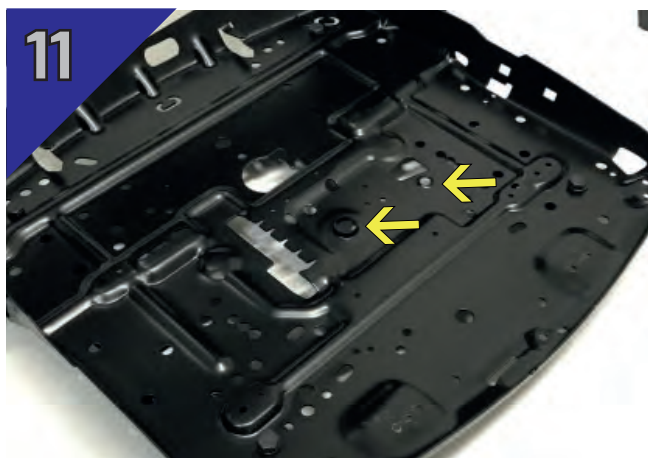
11 Venstre pil viser hull for akseltapp som er rotasjonspunktet mellom svingskive og setetopp. Høyre pil viser hull for montering av låsehendel.
