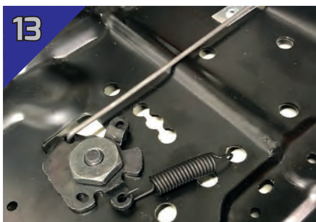
13 Monter fjæren som holder låsehendelen på plass når sving-skiven er i låst posisjon.
